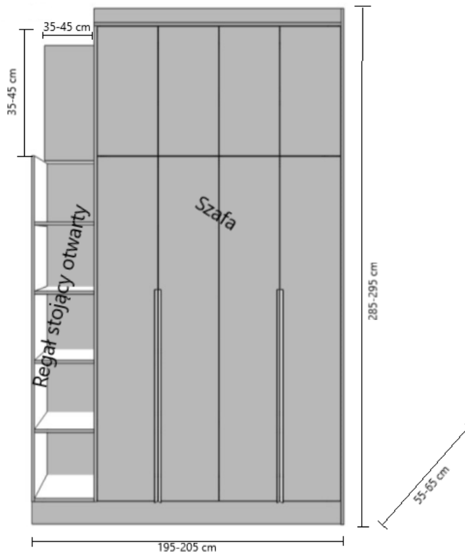
Rzut bok
